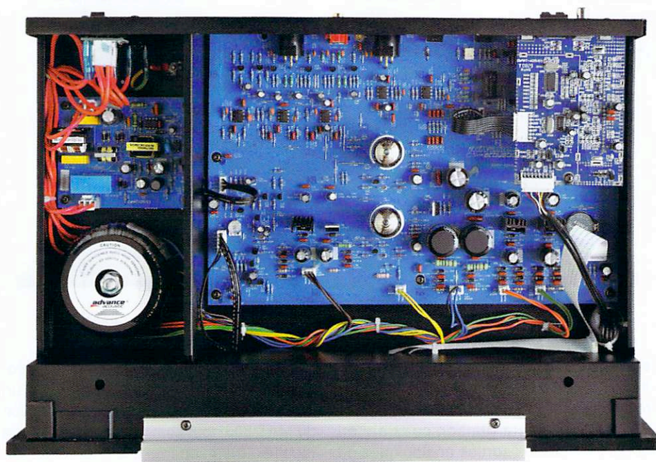
Les deux tubes trônent au centre du grand circuit imprimé du tuner MAT-605
